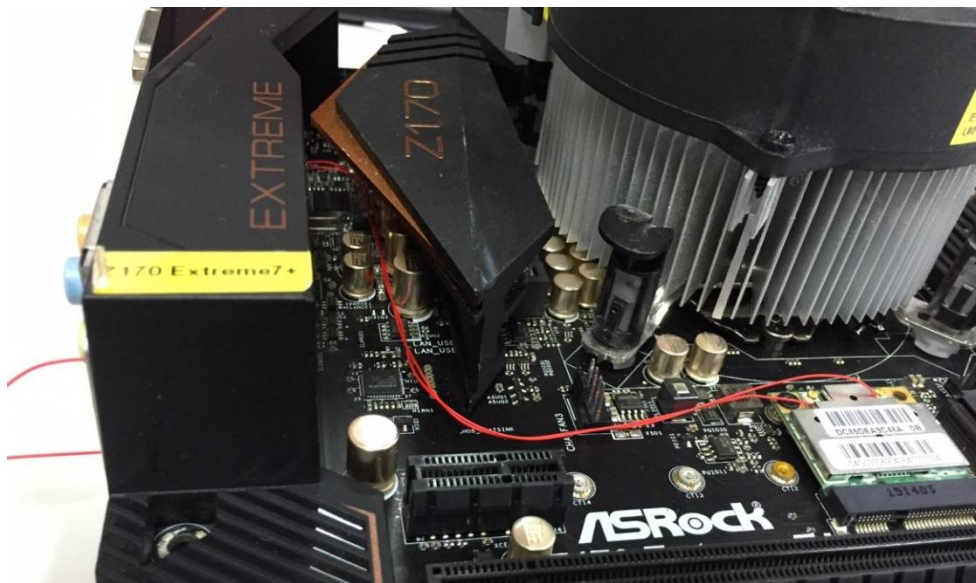
ขั้นที่ 3 - ติดตั้งฝาครอบ IO กลับลงไบน Z170 Extreme7+ ตามรูปด้านล่าง
